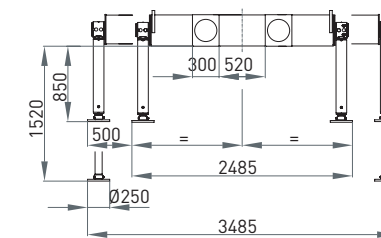
Schwenkabstützung schmal
