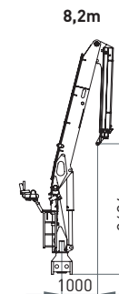
Schwenkabstützung schmal
