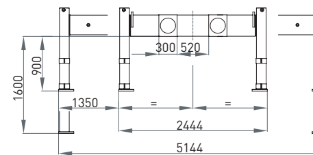
Vierkantabstützung breit
