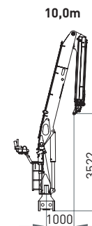
Schwenkabstützung breit
