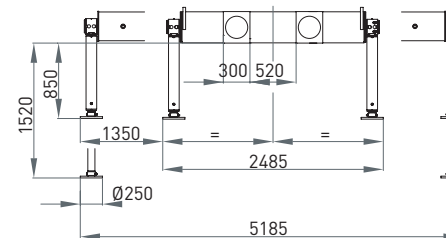
Schwenkabstützung breit
