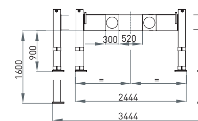
Vierkantabstüttug schmal
